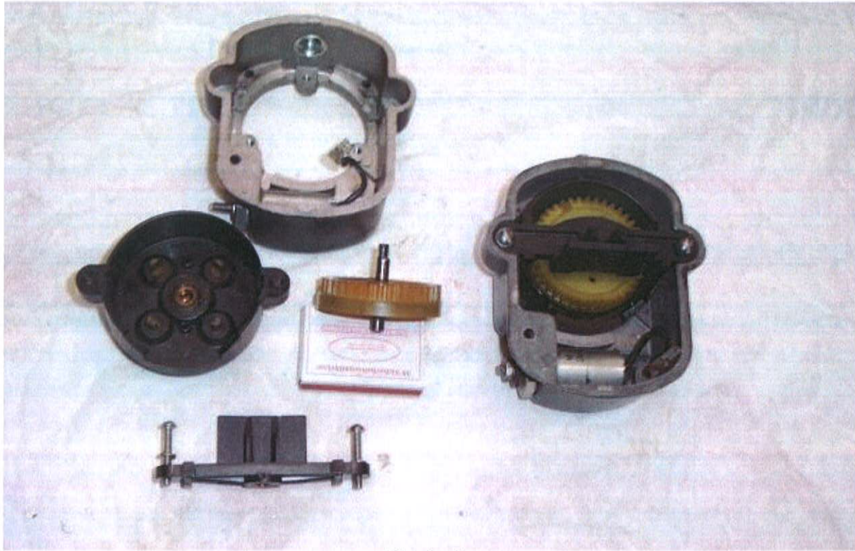
Photo 6: Dis-assembling the distributor drive. Zerlegung des Verteilerantriebes. Démontage du distributeur.
